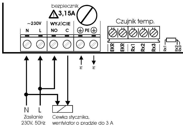
Rys. 2: Schemat połączeń regulatora - sterowanie wentylatora lub cewki stycznika
