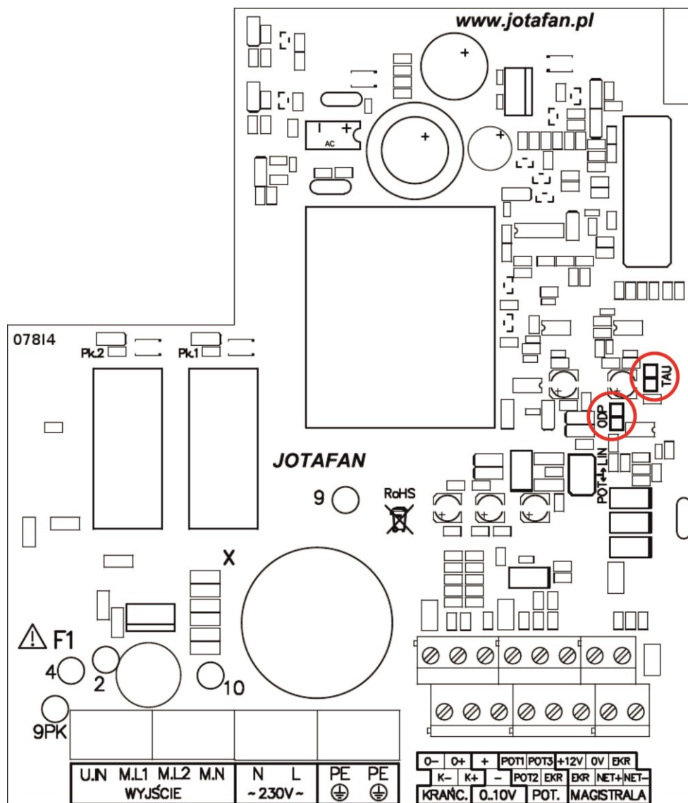
Rysunek 1 Schemat rozmieszczenia elementów na płycie INLET-010-2PK dla wersji PCB 07814.
