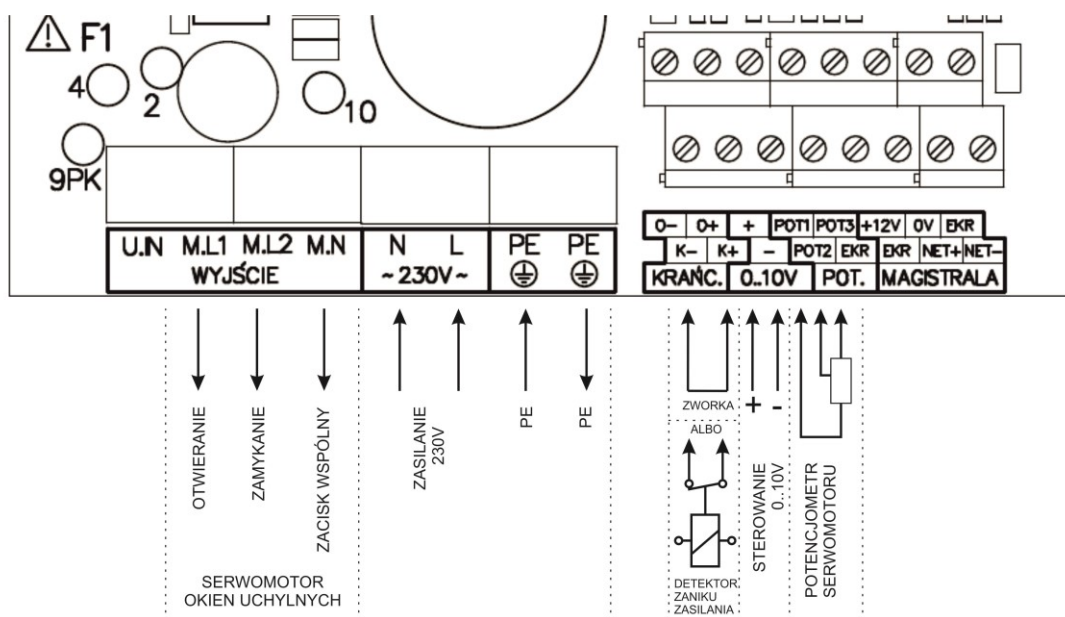
Rysunek 1 Opis zacisków regulatora wlotów INLET-010-2PK przy zadawaniu poziomu otwarcia okien napięciem analogowym 0 .. 10V i wyznaczania aktualnej pozycji okien za pomocą potencjometru serwomechanizmu.
