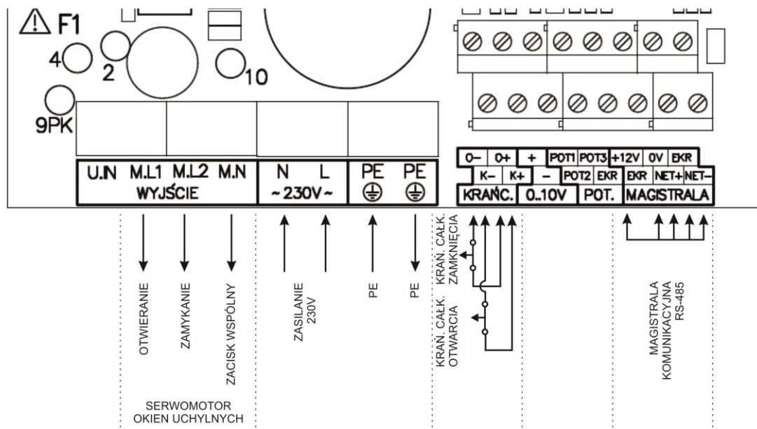
Rysunek 1 Opis zacisków regulatora wlotów INLET-010-2PK przy zadawaniu poziomu otwarcia okien za pomocą interfejsu RS-485 i wyznaczania aktualnej pozycji okien za pomocą pomiaru czasu przejazdu pomiędzy krańcówkami 0% i 100%.
