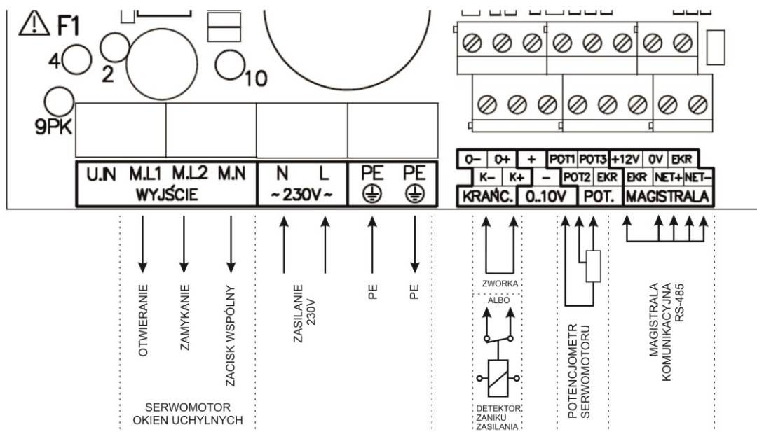
Rysunek 1 Opis zacisków regulatora wlotów INLET-010-2PK przy zadawaniu poziomu otwarcia okien za pomocą interfejsu RS-485 i wyznaczania aktualnej pozycji okien za pomocą potencjometru serwomechanizmu.
