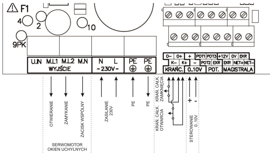
Rysunek 1 Opis zacisków regulatora wlotów INLET-010-2PK przy zadawaniu poziomu otwarcia okien napięciem analogowym 0 .. 10V i wyznaczania aktualnej pozycji okien za pomocą pomiaru czasu przejazdu pomiędzy krańcówkami 0% i 100%.
