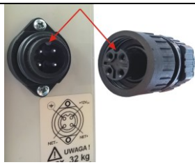
Schemat podłączenia modułu szalki z wtykiem hermetycznym.
