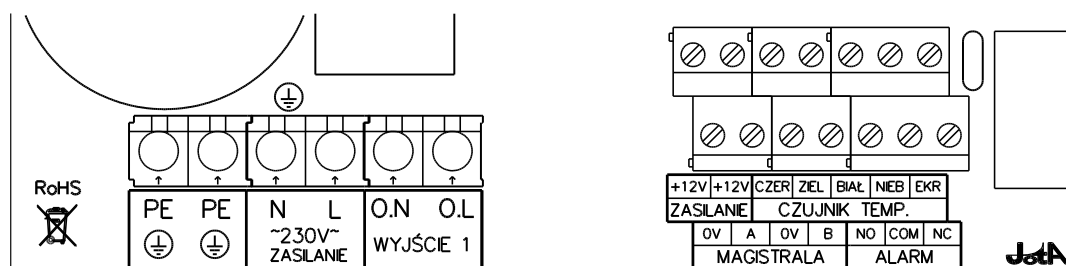
Rysunek 1 Rozmieszczenie zacisków połączeniowych regulatora TERMISTAT-6-AL-010
