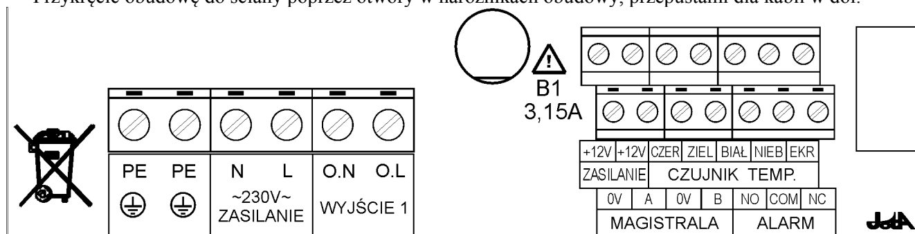
Rys. 1: Rozmieszczenie zacisków połączeniowych regulatora TERMISTAT-6-AL-485
