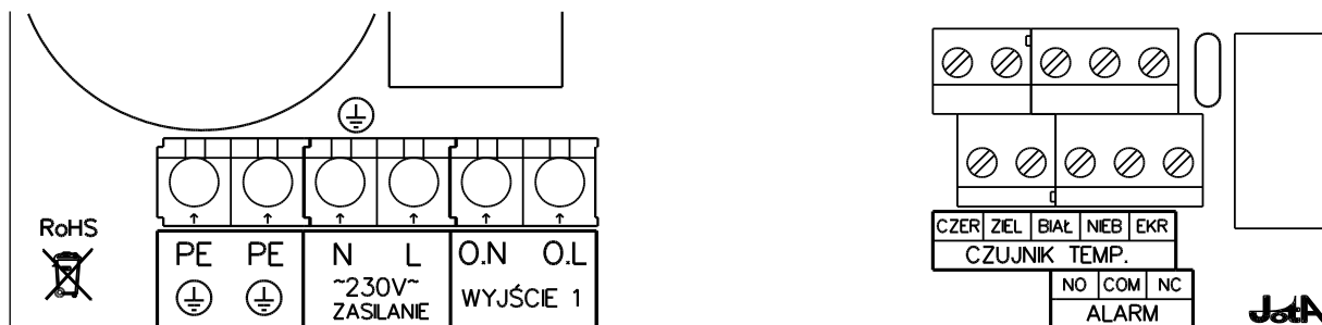
Rysunek 1 Rozmieszczenie zacisków połączeniowych regulatora TERMISTAT-6-AL
